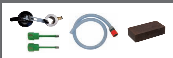
Startset: Anbohrhilfe mit Bohrschablone, Wasserschlauch mit Gardena-Kupplung, Vollbohrkronen 6/8 mm, Schärfstein
