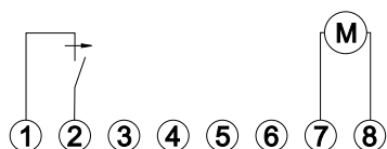
k-Schaltbild
