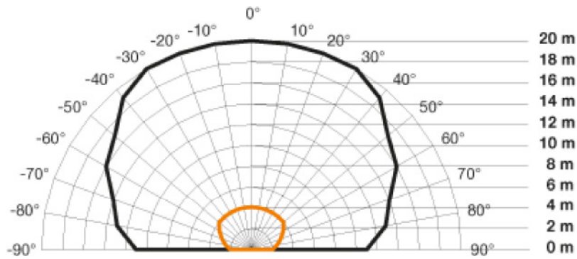
Sensorreichweite IS 2180-5, 20 m Linse
